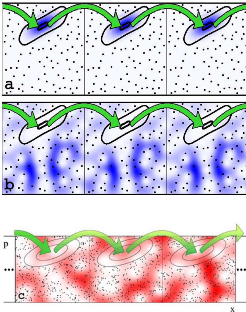
Abb. 3 : Für ein einfaches Modell einer Hamiltonschen Ratsche werden typische quantisierte Zustände mit den invarianten Mengen des klassischen Phasenraumes verglichen. In diesem Fall handelt es sich dabei nur um eine periodische Kette transportierender Inseln, die in die entgegengesetzt transportierende chaotische See eingebettet ist.
