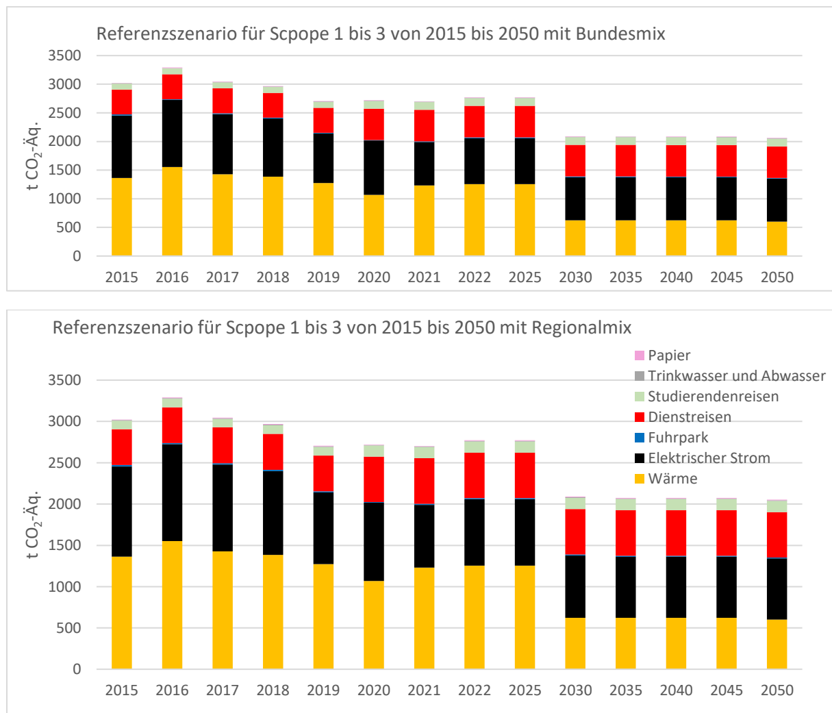
Abbildung 23: Referenzszenario für Scope 1 bis 3 von 2015 bis 2050 mit dem Bundesmix (oben) und dem Regionalmix (unten)
