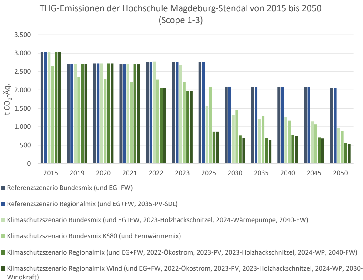
Abbildung 25: Szenarien der THG-Emissionen der Hochschule Magdeburg-Stendal von 2015 bis 2050 (Scope 1-3)
