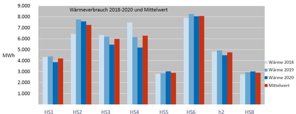
Abbildung 16: Absoluter Wärmeverbrauch von acht deutschen Hochschulen zwischen 2018 und 2020 und Mittelwert (HIS-HE 2022)
