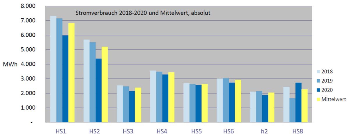
Abbildung 14: Absoluter Stromverbrauch von acht deutschen Hochschulen zwischen 2018 und 2020 und Mittelwert (HIS-HE 2022)
