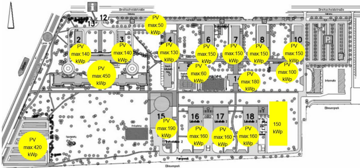
Abbildung 30: Potenziale für die Stromerzeugung auf dem Campus Herrenkrug für PV mit der Annahme, dass eine 1-kWp-Anlage jährlich 1 MWh erzeugt (ITG 2017).
