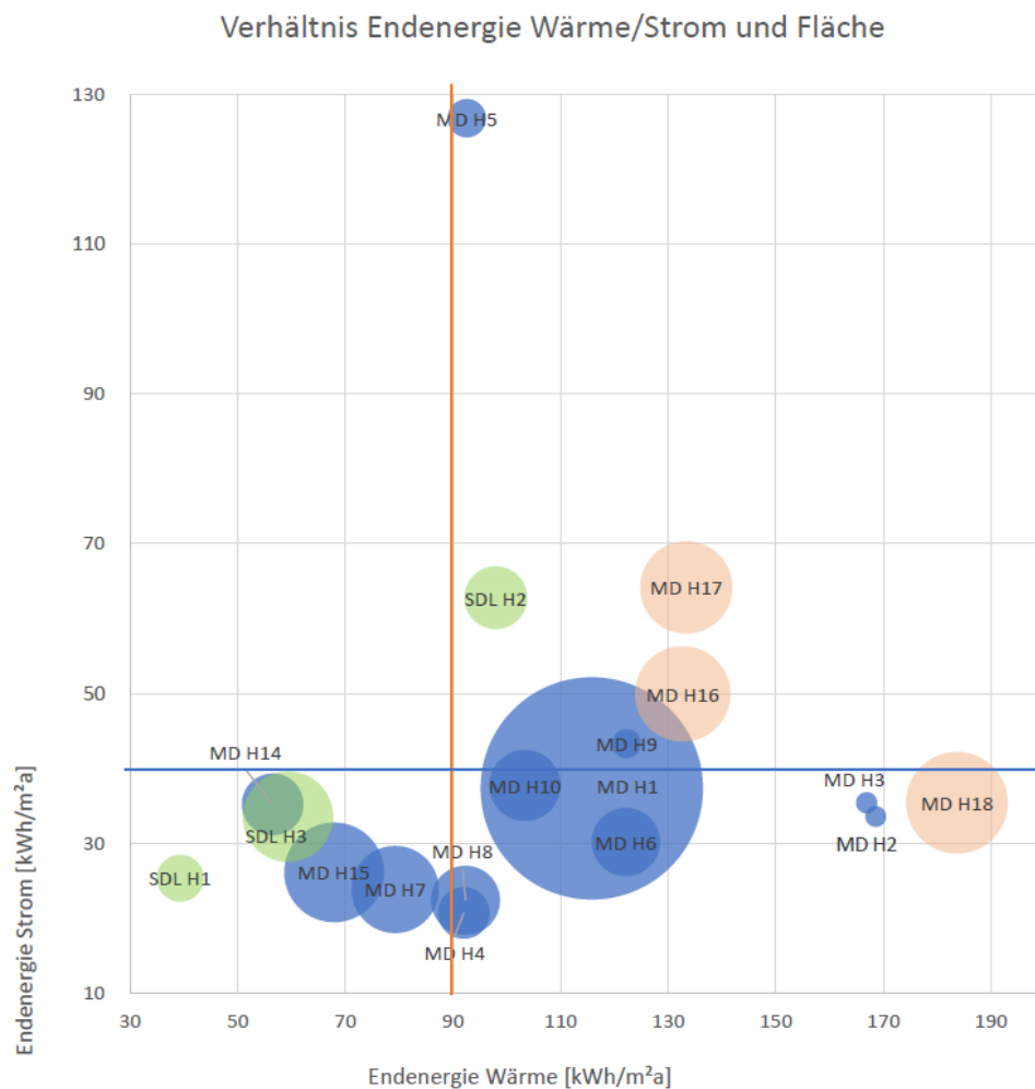
Abbildung 28: Verhältnis Endenergie Wärme/Strom und Fläche: Stendal: grün, blau: Büro- und Schulungsbauten, orange: Laborhallen (STEINWENDER ET AL. 2023).
