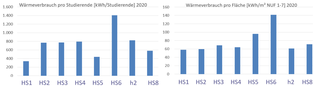
Abbildung 17: Stromverbrauch pro Studierende und pro Fläche (NUF 1-7) von acht deutschen Hochschulen 2020 (HIS-HE 2022)
